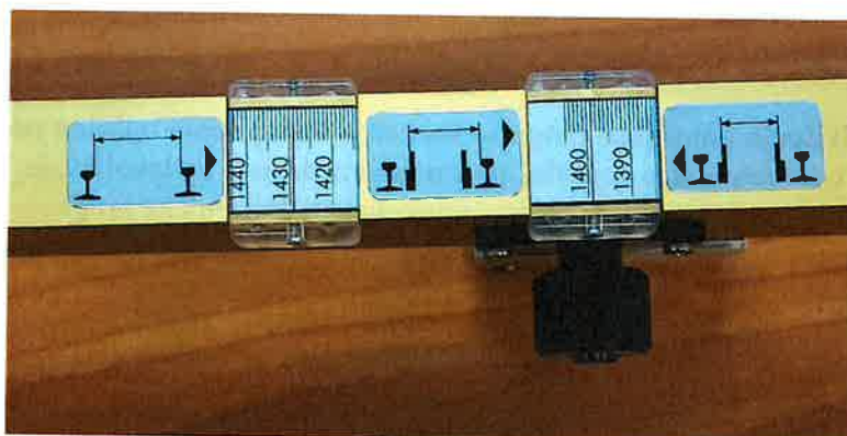
Slika 2. Uredaj za ispitivanje širine kolosijeka
